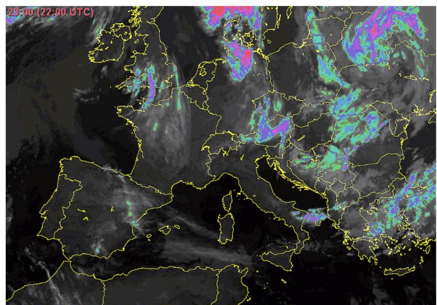
Date: 28/12/16. Image fournie par Sat24.com sur la base des données Eumetsat / DWD / N O. Colorisée par www.meteo60.fr. Légende sur www.meteo60.fr
