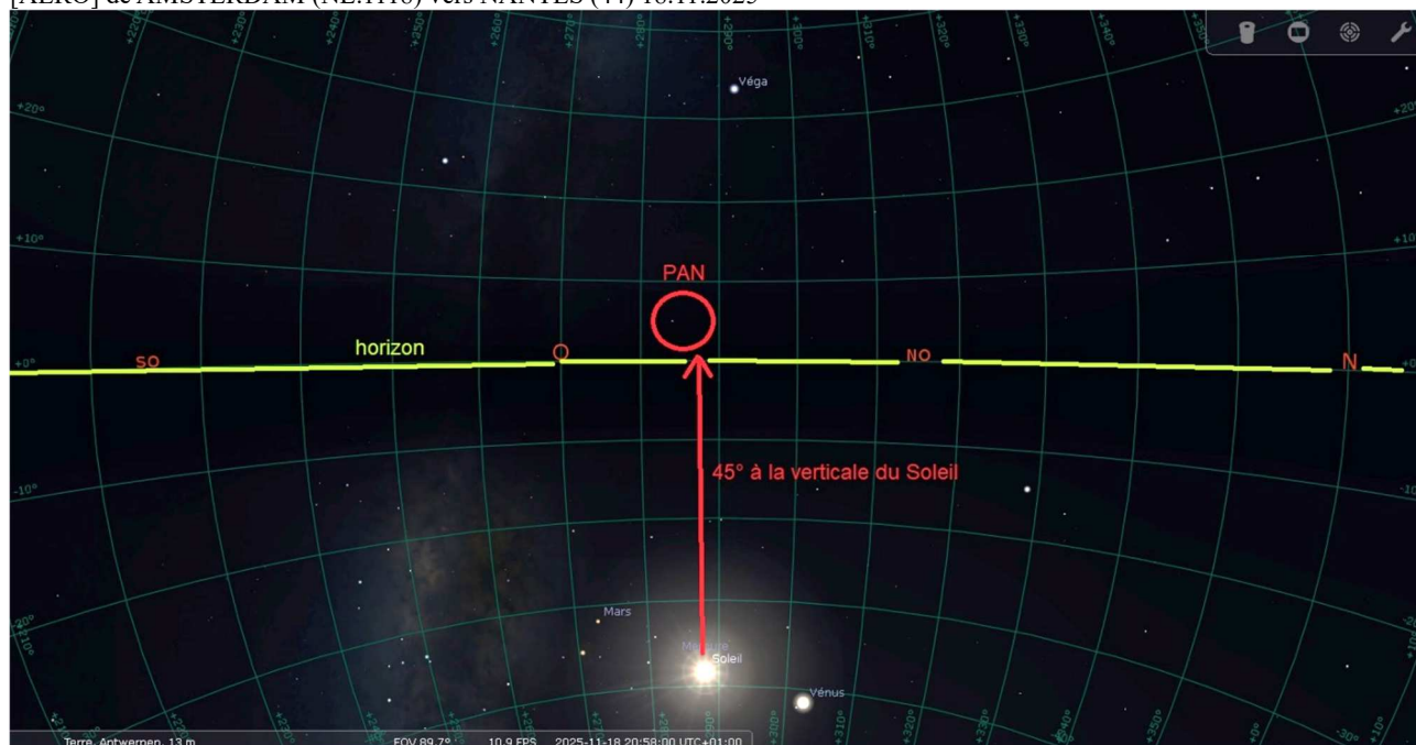
Reconstitution de la position du PAN par rapport au Soleil à 20h58 le 18/11/2025 (image : Stellarium)
